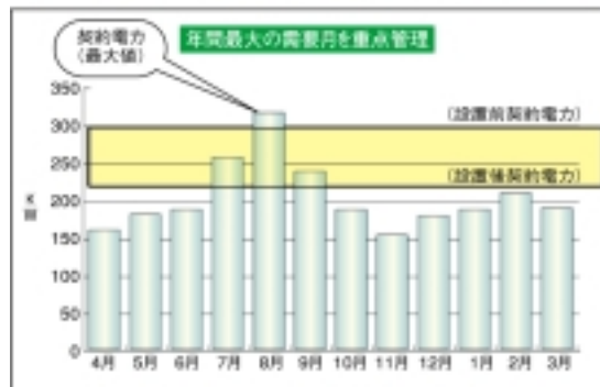
デマンド監視装置設置によるピークカットのイメージ
